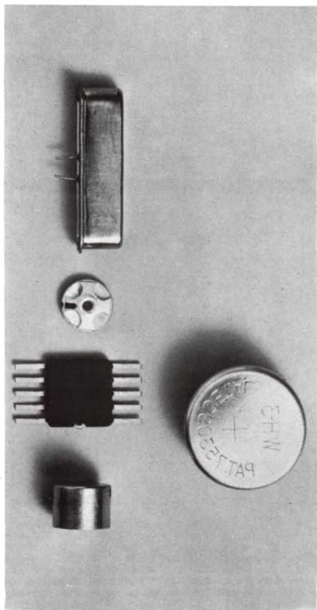
Studiati sulla base del nuovo motore passo-a-passo Socrem S 05, ecco gli elementi elettronici che permettono di costruire un orologio a quarzo. (PORTESCAP).
