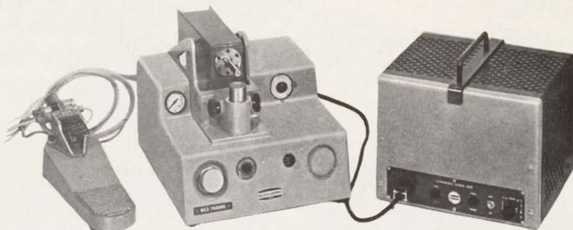
FIG. 8 - Saldatrice ad ultrasuoni tipo SL 86 per materiali metallici.
