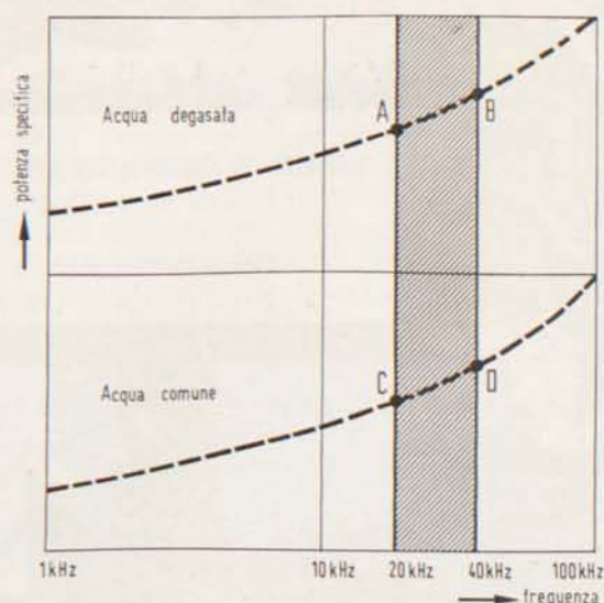
Diagramma 1. - Potenze in W/cm^2 necessarie a produrre cavitazione nel mezzo liquido per frequenze variabili fra 1 kHz e 100 kHz. Entrambe le coordinate sono in scala logaritmica. I valori dei punti segnati sono, in W/cm^2 : A = 12; B = 16; C = 1.2; D = 1.6.
