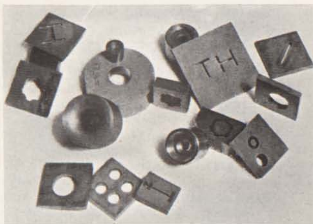
FIG. 7 - Lavorazioni realizzate col trapano ad ultrasuoni in materiali duri e fragili.
