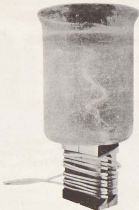
FIG. 2 - Complesso di dimostrazione che permette di osservare gli effetti della cavitazione.
