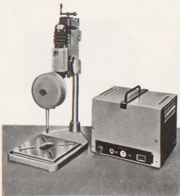
FIG. 5 - Trapano ad ultrasuoni della potenza di 60W
