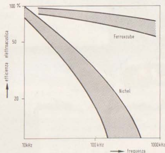
Diagramma 2. - Diagrammi frequenza — efficienza elettroacustica relativi a trasduttori in ferroxcube e in nickel. Dal raffronto risulta evidente la più elevata efficienza elettroacustica propria del ferroxcube nell'intera banda di frequenza.
